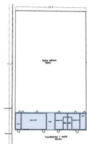
Plan du bâtiment
